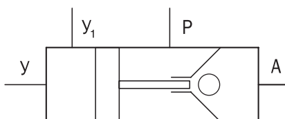
Схема гидравлическая принципиальная для П786Б
